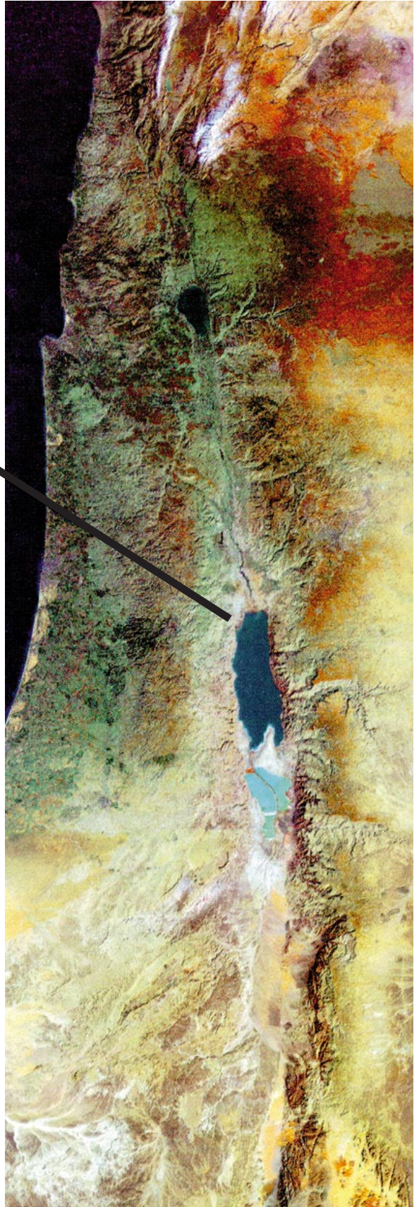
Fotografías del Lago de Lot tomadas desde un satélite.
