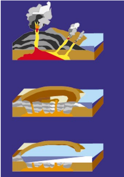
Ilustración que muestra la erupción volcánica y el colapso que se produjo a continuación, el cual motivó la desaparición de todo el pueblo.
