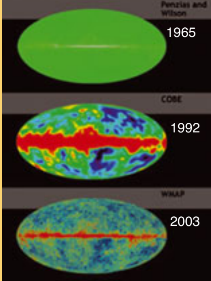
Penzias ve Wilson'ın keşfettiği Kozmik Fon Radyasyonu, Big Bang'in kesin bir delili olarak bilim tarihine geçti.
