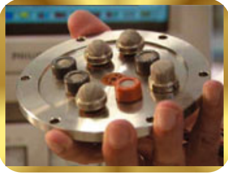
(Şekil 21) Elektronik burunda kullanılan bazı sensörler. Bu sensörler, koku alma sistemindeki reseptörlerden ilham alınarak tasarlanmıştır; bununla birlikte insan burnundaki reseptörlerle kıyaslanmayacak kadar ilkelidirler.
