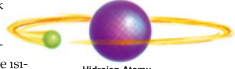
Hidrojen Atomu
