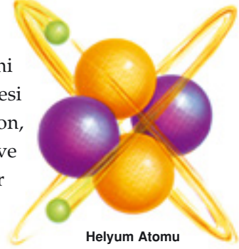
Helyum Atomu
